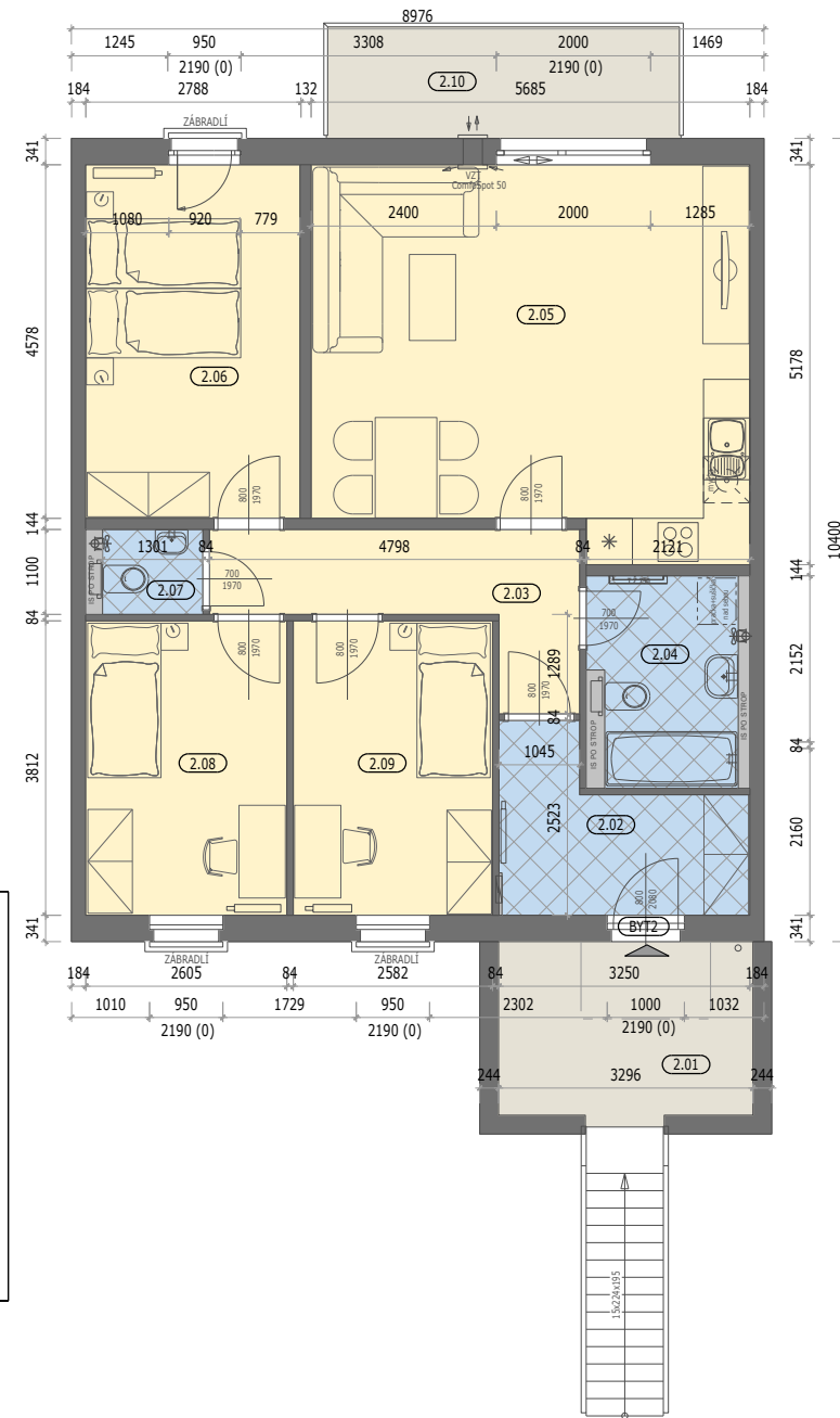
místnost účel miestnosti plocha m 2 podlahovina 2.02 ZADVERI 6,00 DREVO 2.03 CHODBA 6,60 LAMINO 2.04 KOUPELNA 5,10 DLAŽBA 2.05 OBYVACI POKOJ + KUCHYŇ 27,30 LAMINO 2.06 POKOJ 12,70 LAMINO 2.07 WC 1,40 DLAŽBA 2.08 POKOJ 10,00 LAMINO 2.09 POKOJ 9,90 LAMINO
